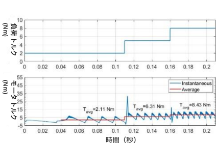
図2. 負荷トルクに対するモータトルクの変化 (シミュレーション結果) 本発明の制御方法を行った場合、負荷トルクの増加に対して、モータトルクの増加率が高いことから、効率が約10~20%増加した。
