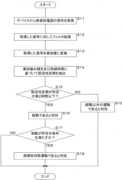
図2 処理フローチャート 第2時間は図1のTdを指す
