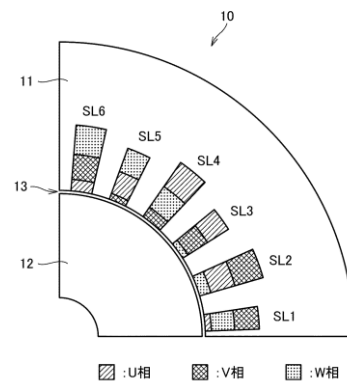
図2 スロット内の巻線配置の例
