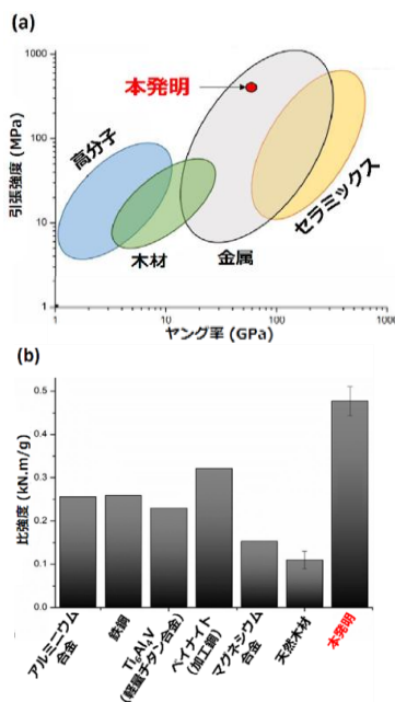
図3. 既存材料との強度比較
