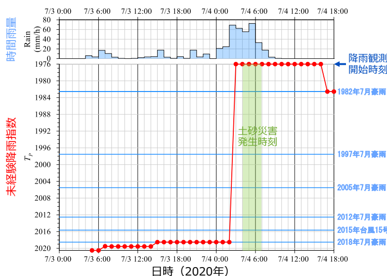
図 1. 2020年7月豪雨における戸北町(熊本)の未経験降雨指数の時間変化
