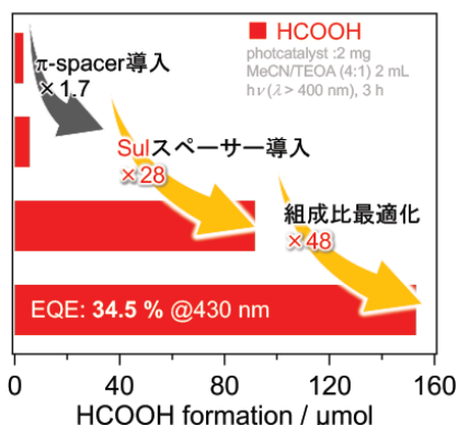
図2. 本発明における設計の最適化による光利用効率の向上
