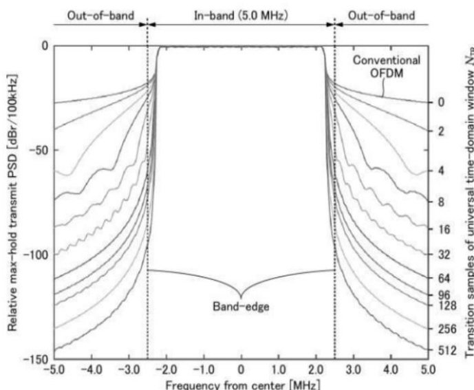
図1 LTE信号を用いた計算機シミュレーションにより帯域外輻射電力抑圧性能の評価 時間軸ウィンドウイング処理を全く施さない場合(窓遷移長 N_{TR} = 0 : 従来例)の場合には、帯域外においてスペクトラムマスク(所定の基準値)を超える周波数成分が大きいものに対して、時間軸ウィンドウイング処理(本件発明)を施した場合には、OFDM信号の帯域外の輻射電力が抑圧される。
