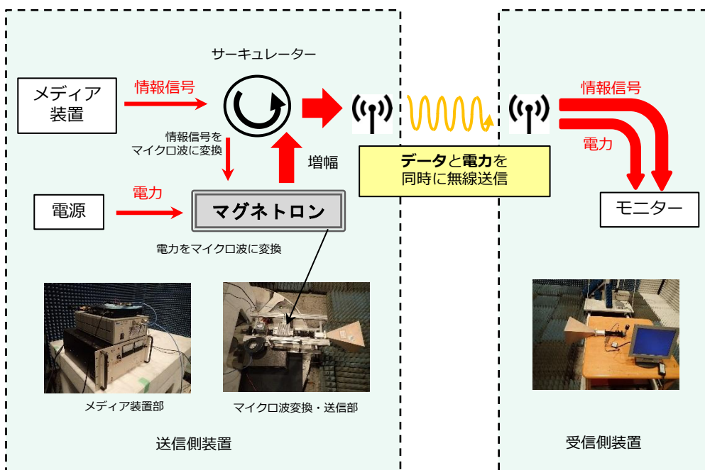
図. 本発明のマイクロ波送信装置の概略
